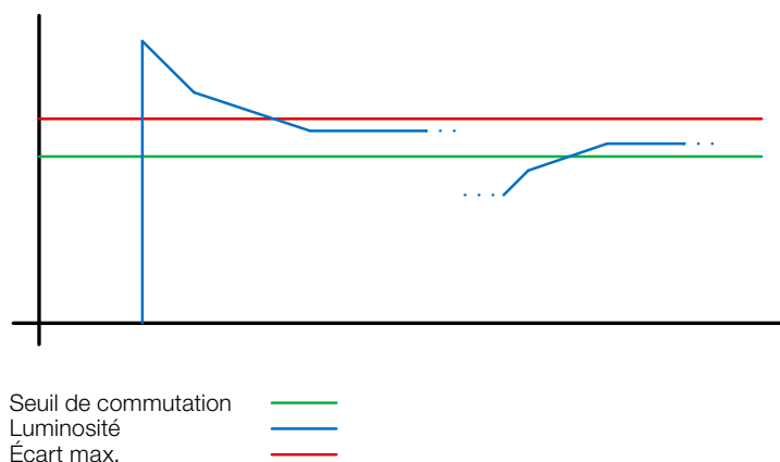
Figure 3 : correction de la plage maintien d'un éclairage constant
